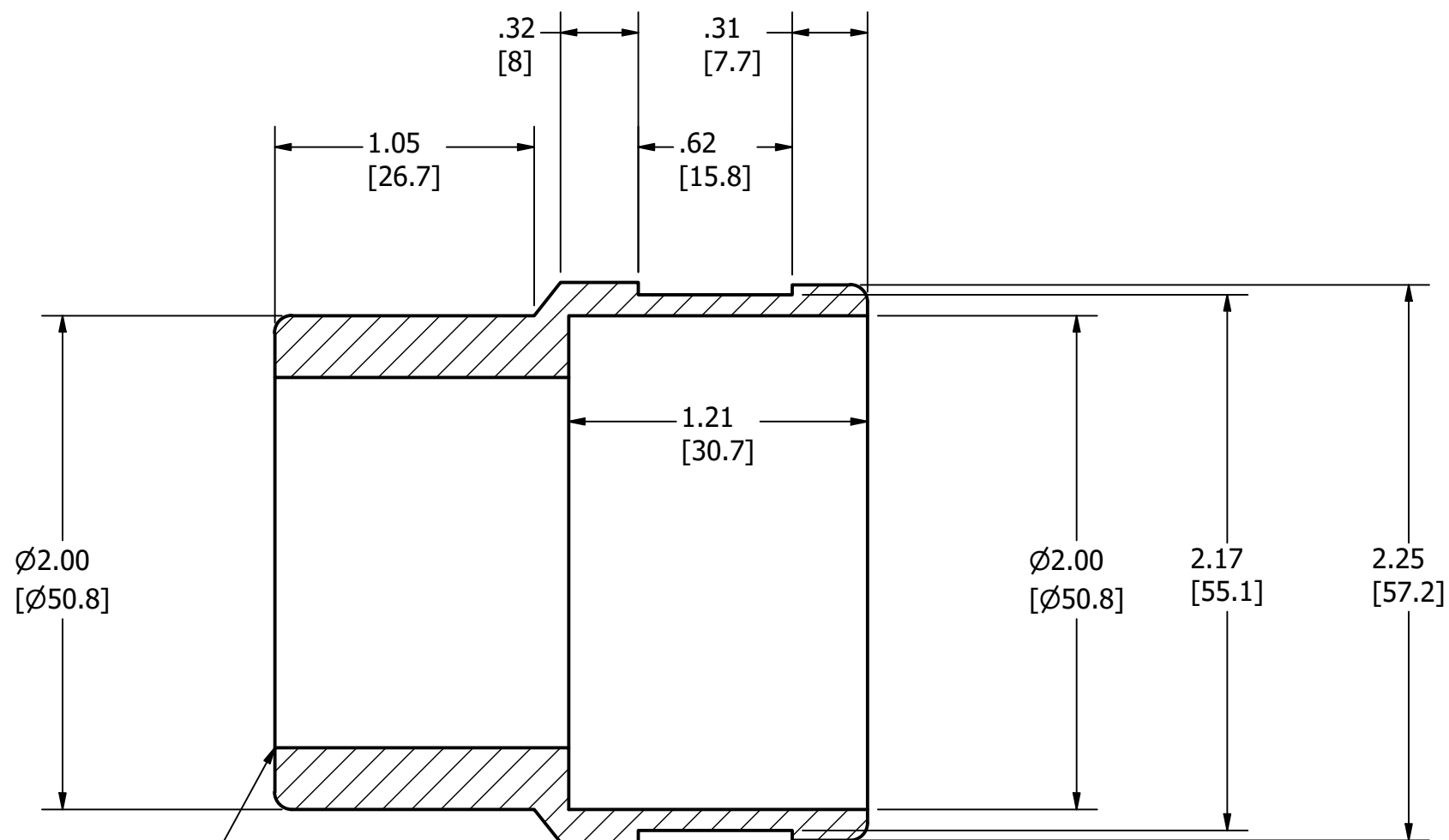
SECTION A-A SCALE 1.5 : 1
