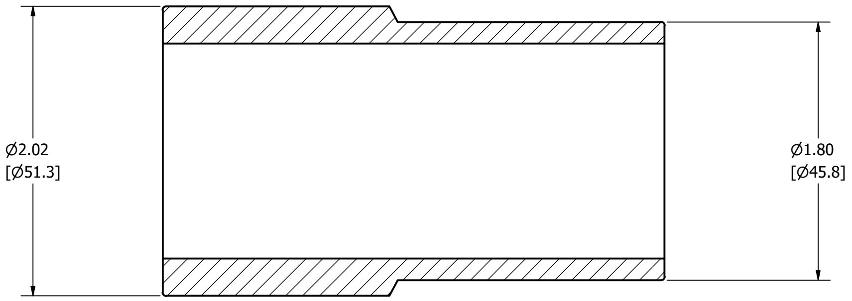
SECTION A-A SCALE 1.5 : 1
