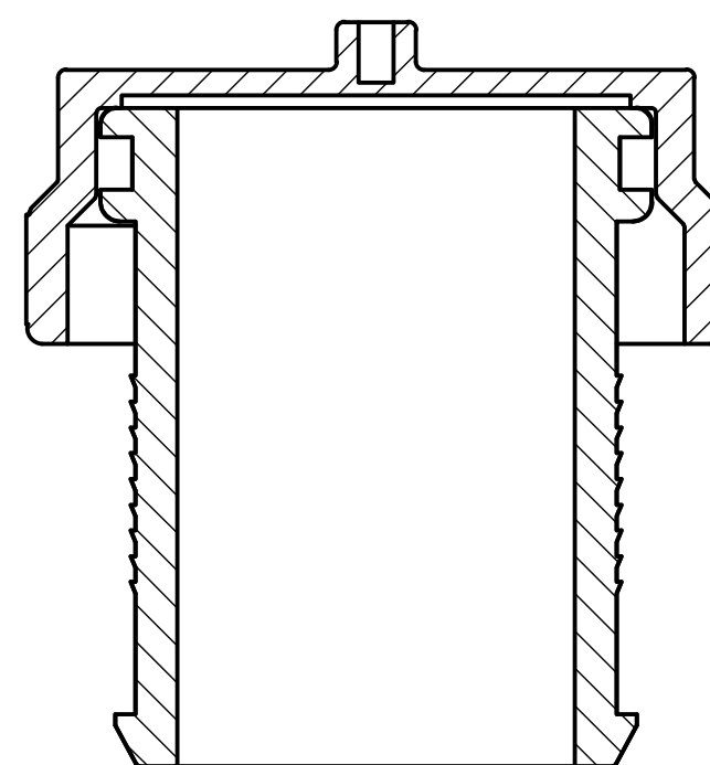
SECTION A-A SCALE 1.5 : 1
