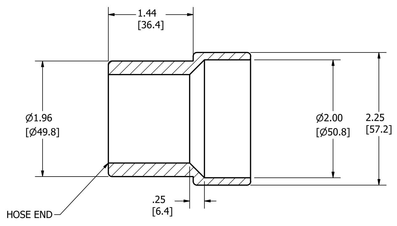
SECTION A-A SCALE 1 : 1
